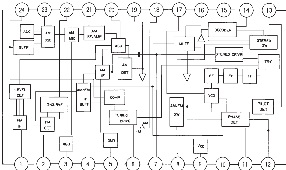
IC102 LA1831
